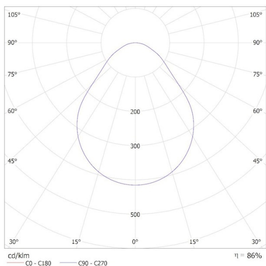
KANLUX S.A. (kat 26759) AVAR U 6262 32W-CCT / Krzywa rozsyłu światła (biegunowo)
